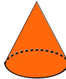
Cone
